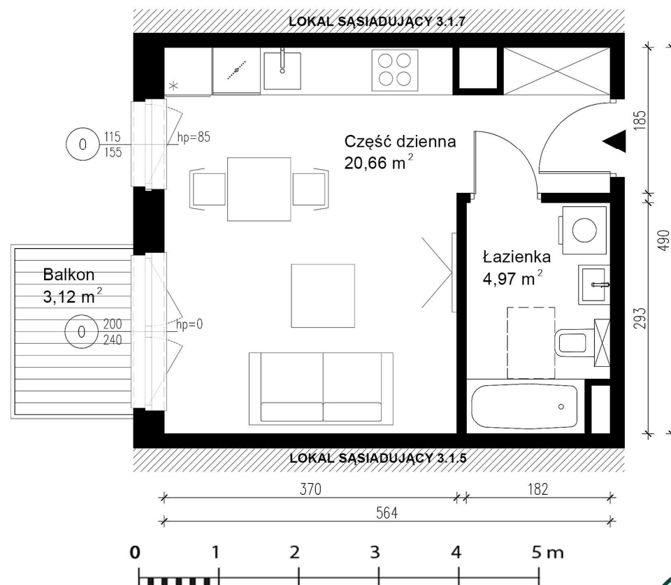
Rzut 1. piętra
