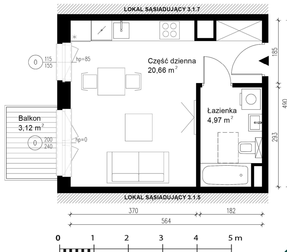
Rzut 1. piętra
