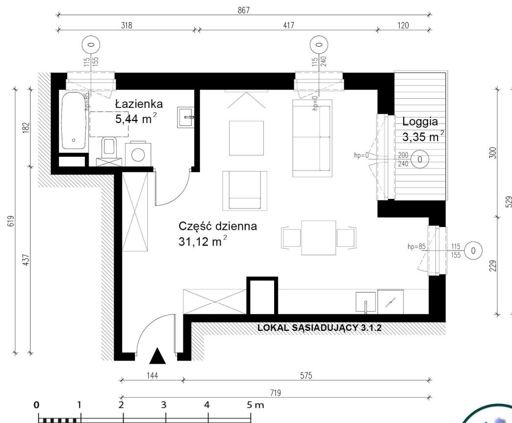
Rzut 1. piętra
