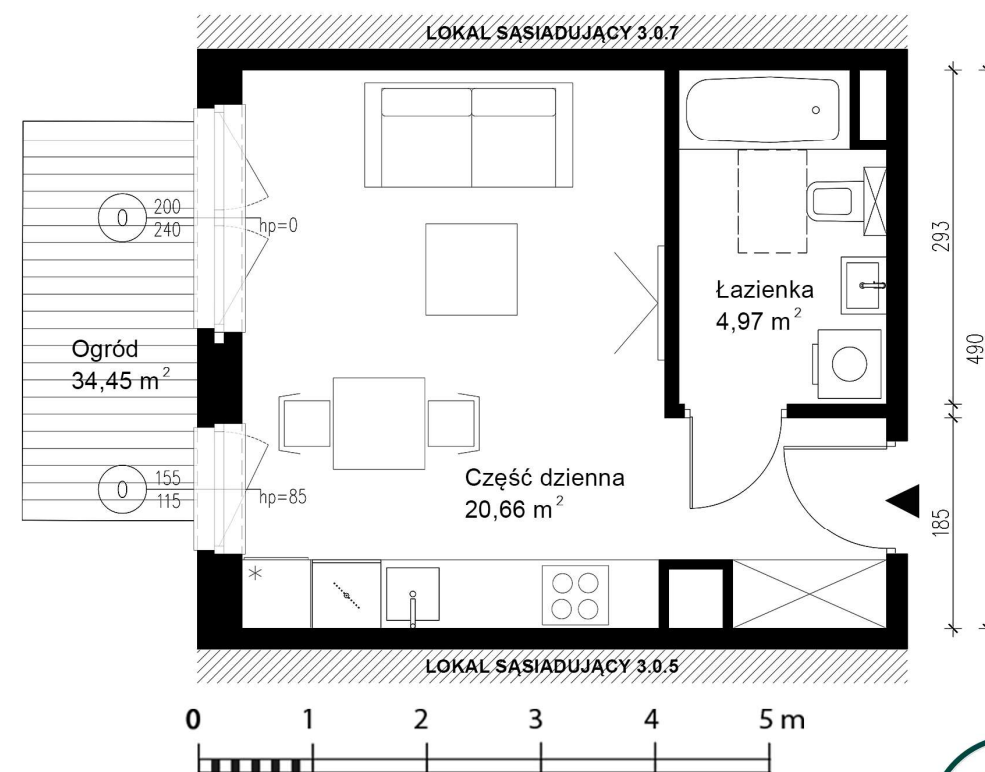
Rzut parteru
