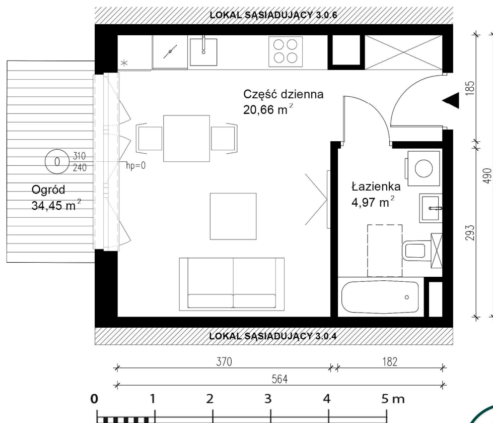
Rzut parteru
