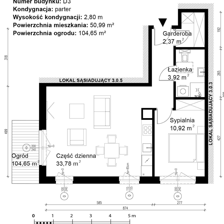
Rzut parteru
