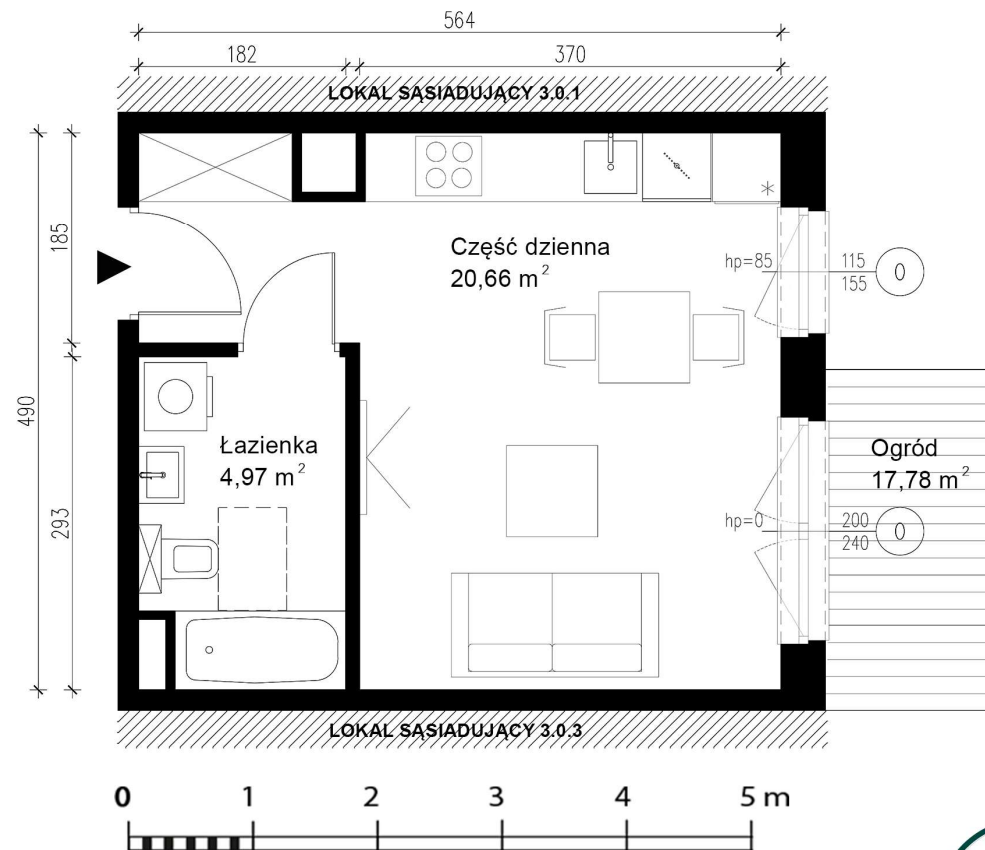
Rzut parteru
