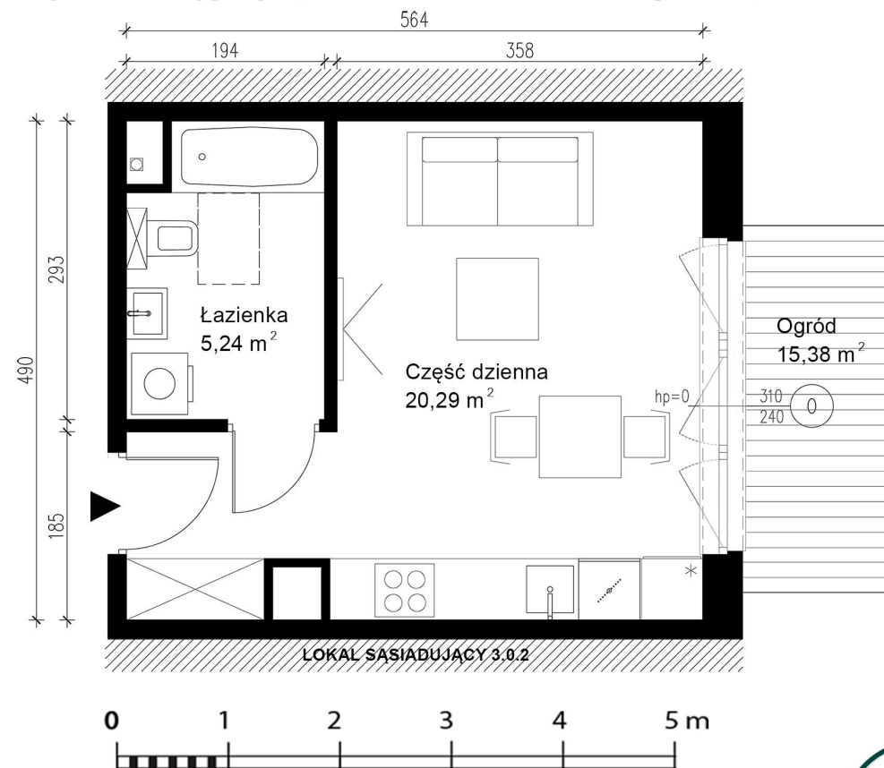
Rzut parteru
